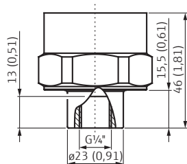
Rosca ISO 228 G \frac{1}{4} " (hembra)
