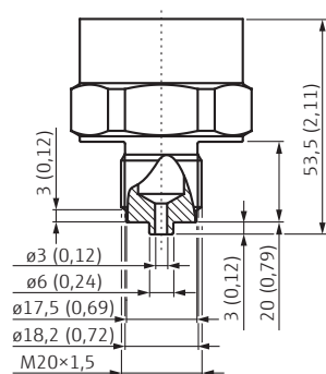
Rosca DIN13
