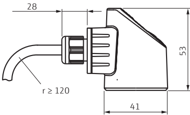
Cable
