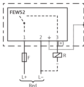
Conexión de la electrónica FEW52
