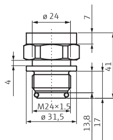
Rosca M24×1,5
