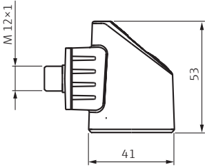
Conector M12, Cubierta de la caja de plástico
