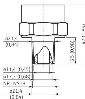
ASME \frac{1}{2} " MNPT, orificio 11,4 mm (0,45 pulgadas)
